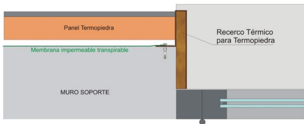
Esquema de instalación de un recerco térmico para Termopiedra
